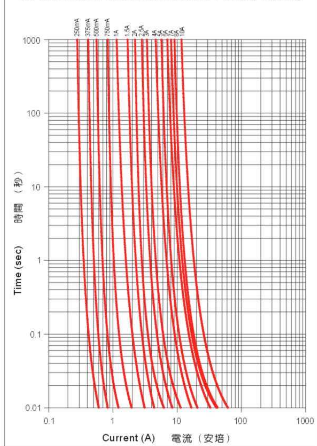
3FP Time-Current Characteristic Curves 平均時間-電流曲線
